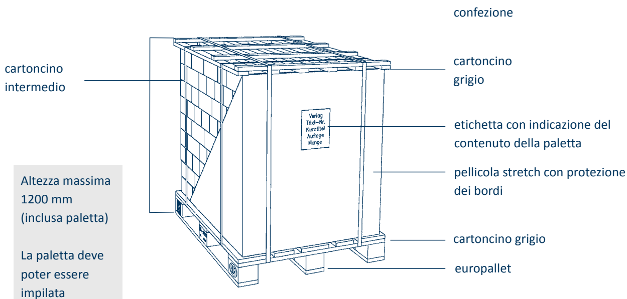
Figura: consegna di una paletta imballata
